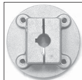
Fan Hub TK P/N 77-1457 Carrier P/N 20-77-1457
